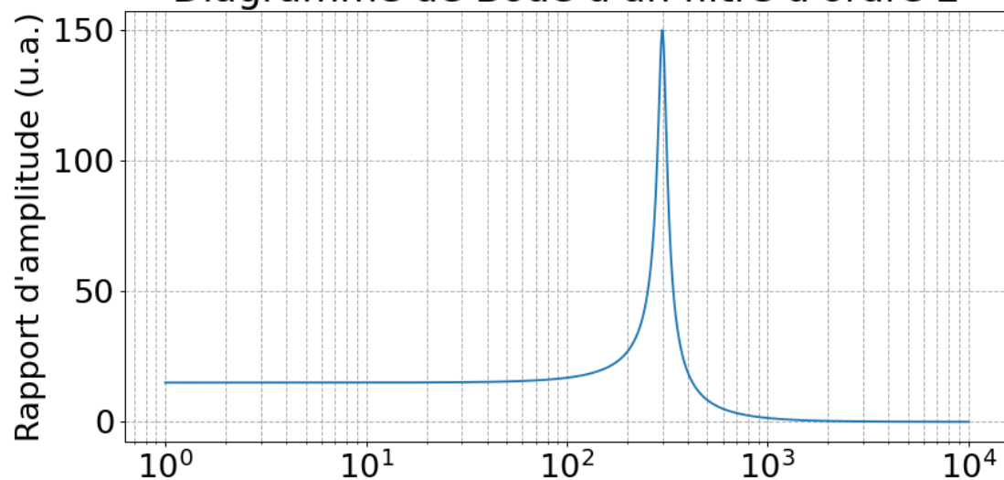
Diagramme de Bode d'un filtre d'ordre 2
