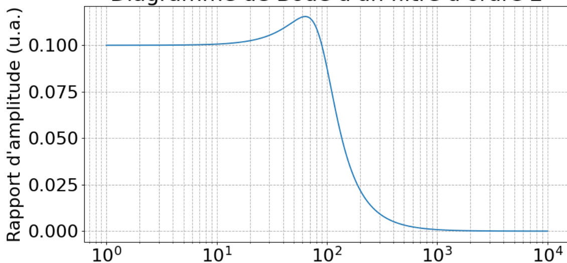
Diagramme de Bode d'un filtre d'ordre 2
